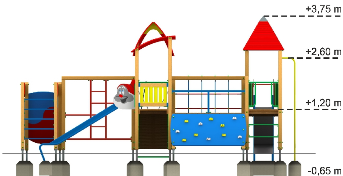
Rys. 4 Zestaw zabawowy duży (widok z boku - z wysokościami).
