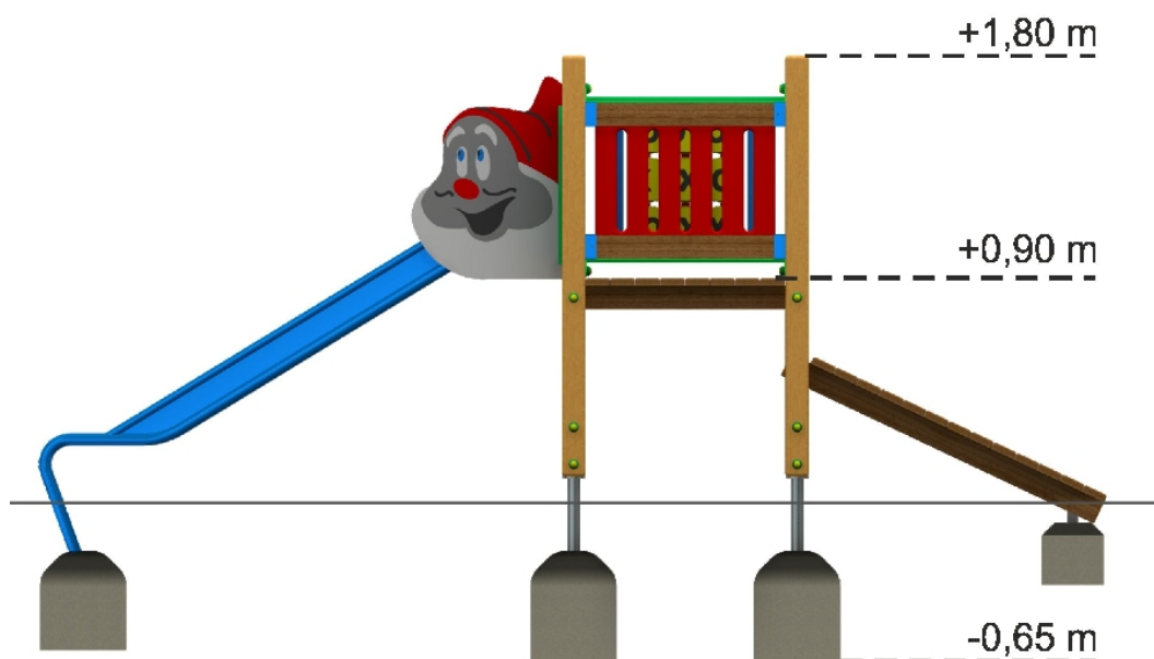
Rys. 6 Zjeżdżalnia mała (widok z boku - z wysokościami).
